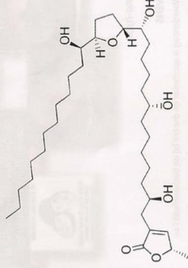
Structuurformule annonacin.
